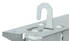
Integrerat linfäste
